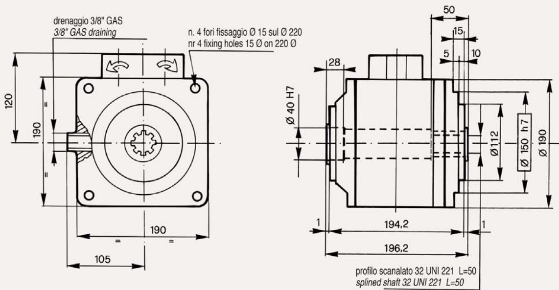
Versione standard con albero cavo Standard version with hollow shaft
